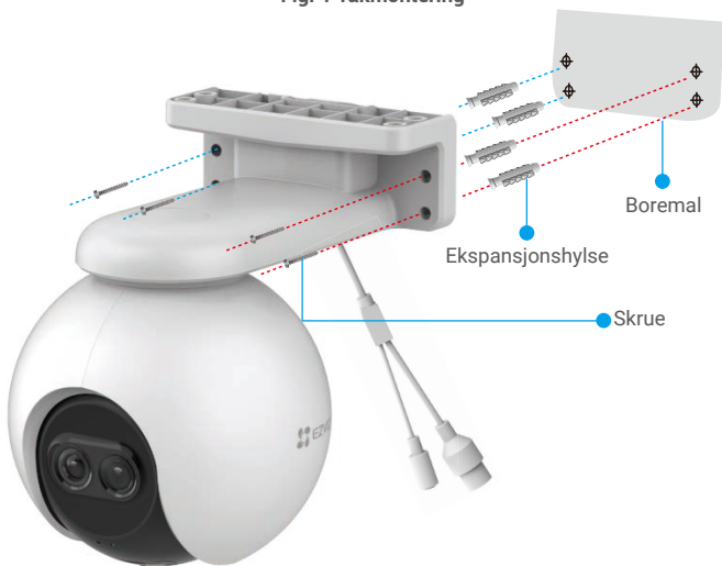
Fig. 2 Veggmontering
