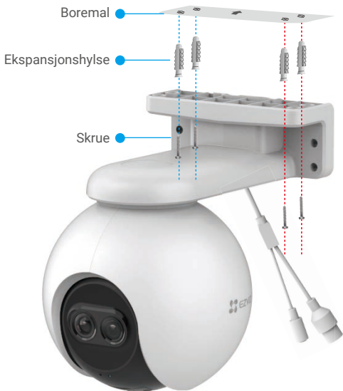
Fig. 1 Takmontering
